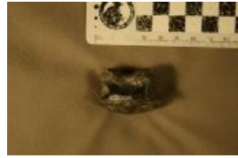
Sauropoda indet. (6967)
